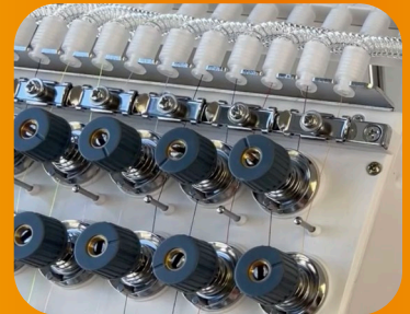
Commandes de réglage de la tension du fil
